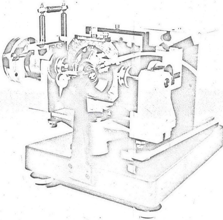
Fig. 2 - Chambre à précession pour les études de diffraction X sous pression
